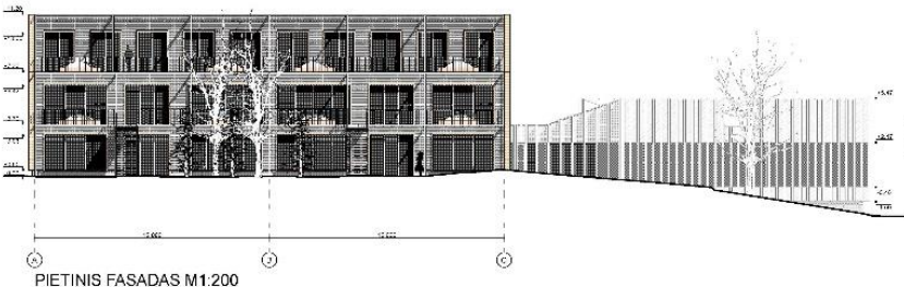
PIETINIS FASADAS M1:200
