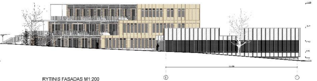
RYTINIS FASADAS M1:200
