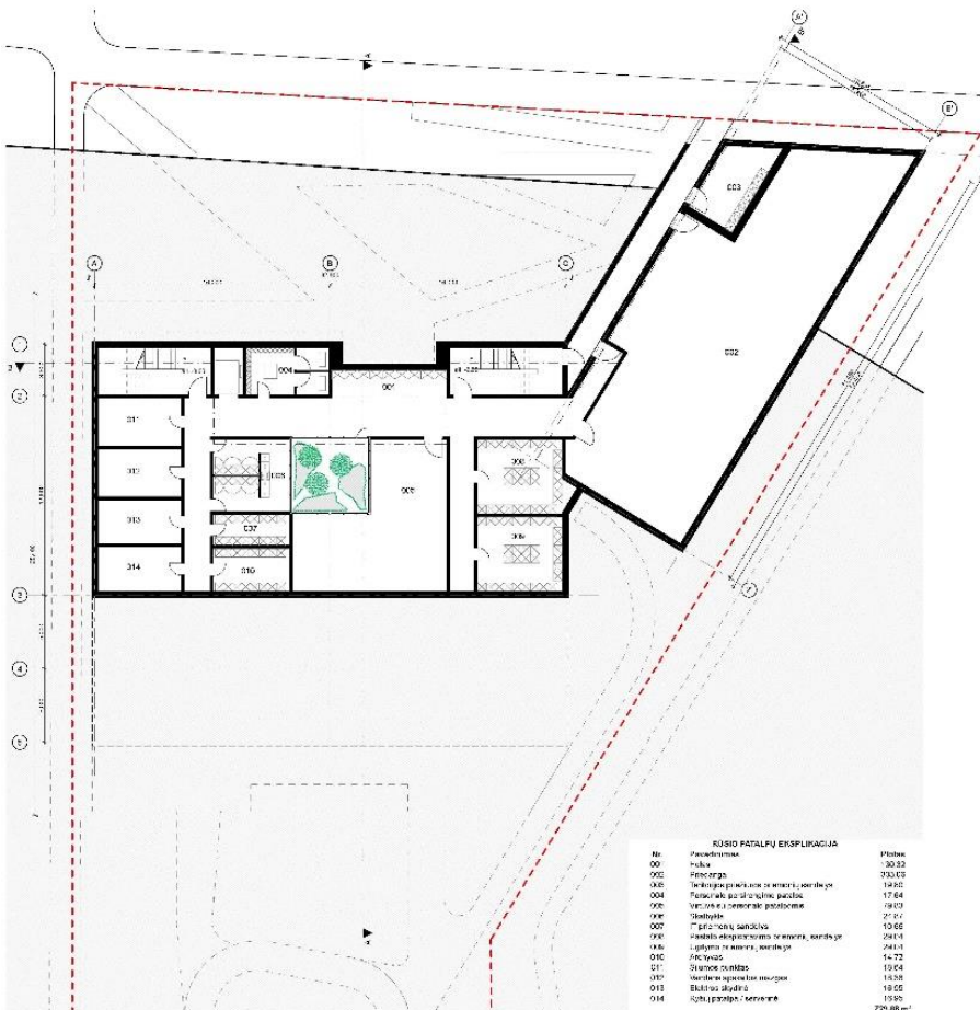
RŪSIO PLANAS M1:200
