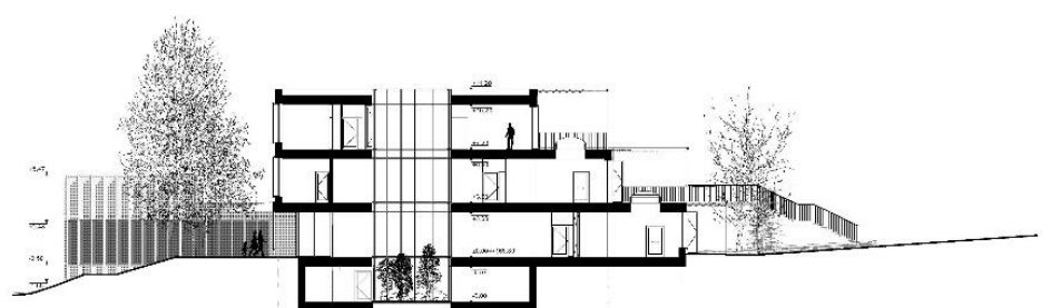
PŪVIO A-A' M1:200
