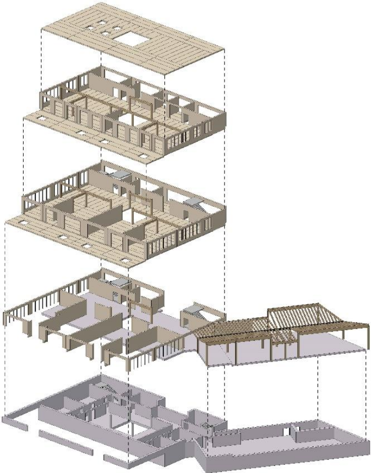
KONSTRUKCINE SCHEMA
