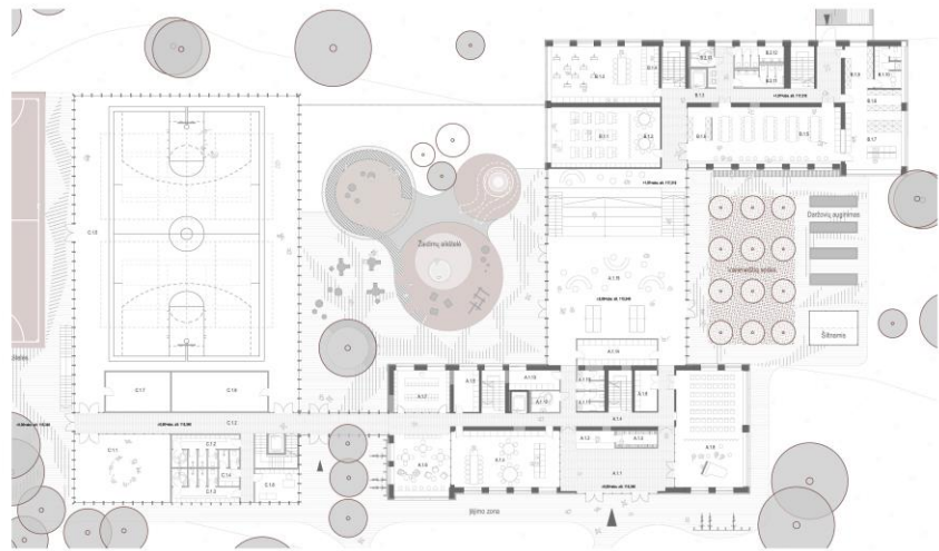
PIRMO AUKŠTO PLANAS, M1:200
