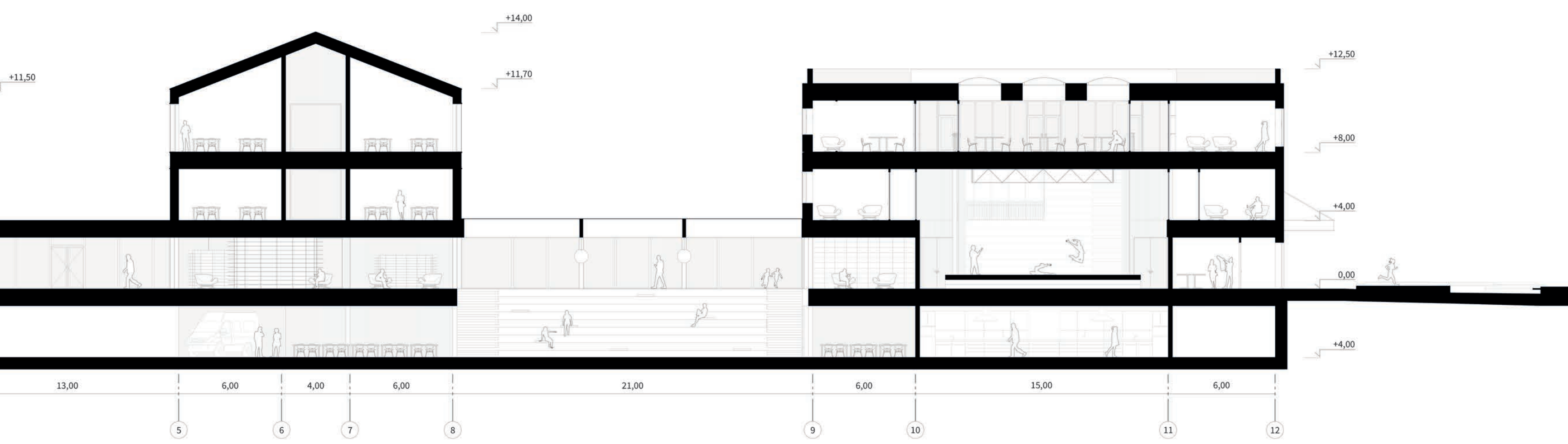
PJŪVIS A-A M 1:200
