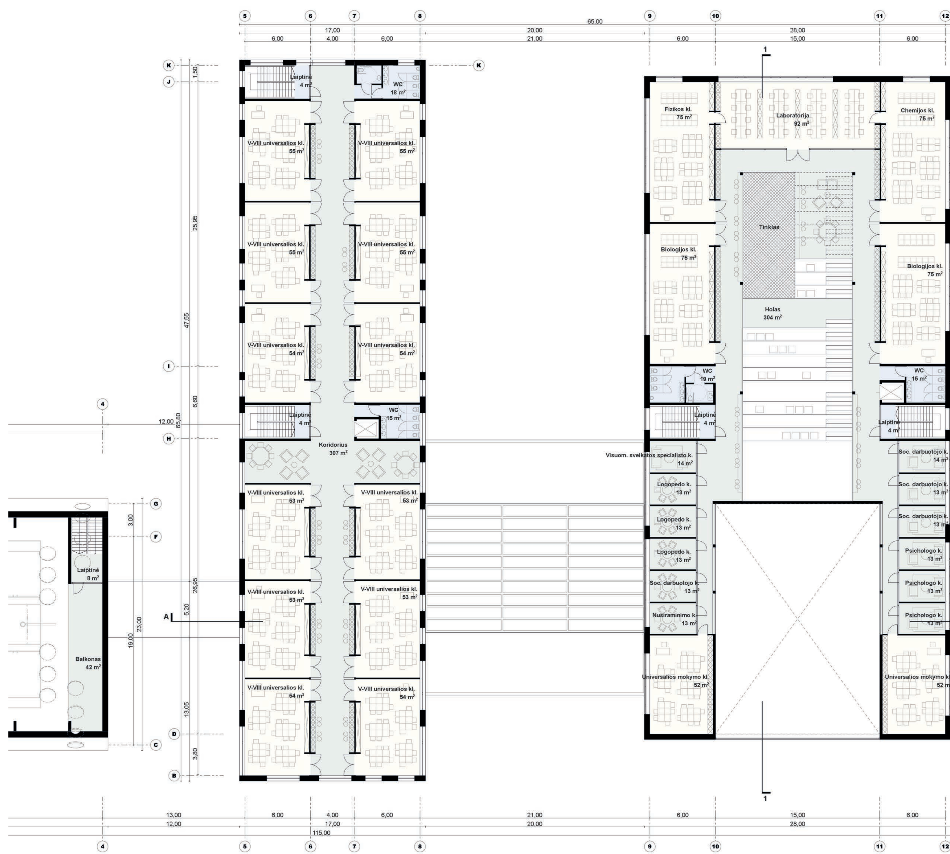
ANTRO AUKŠTO PLANAS M 1:200
