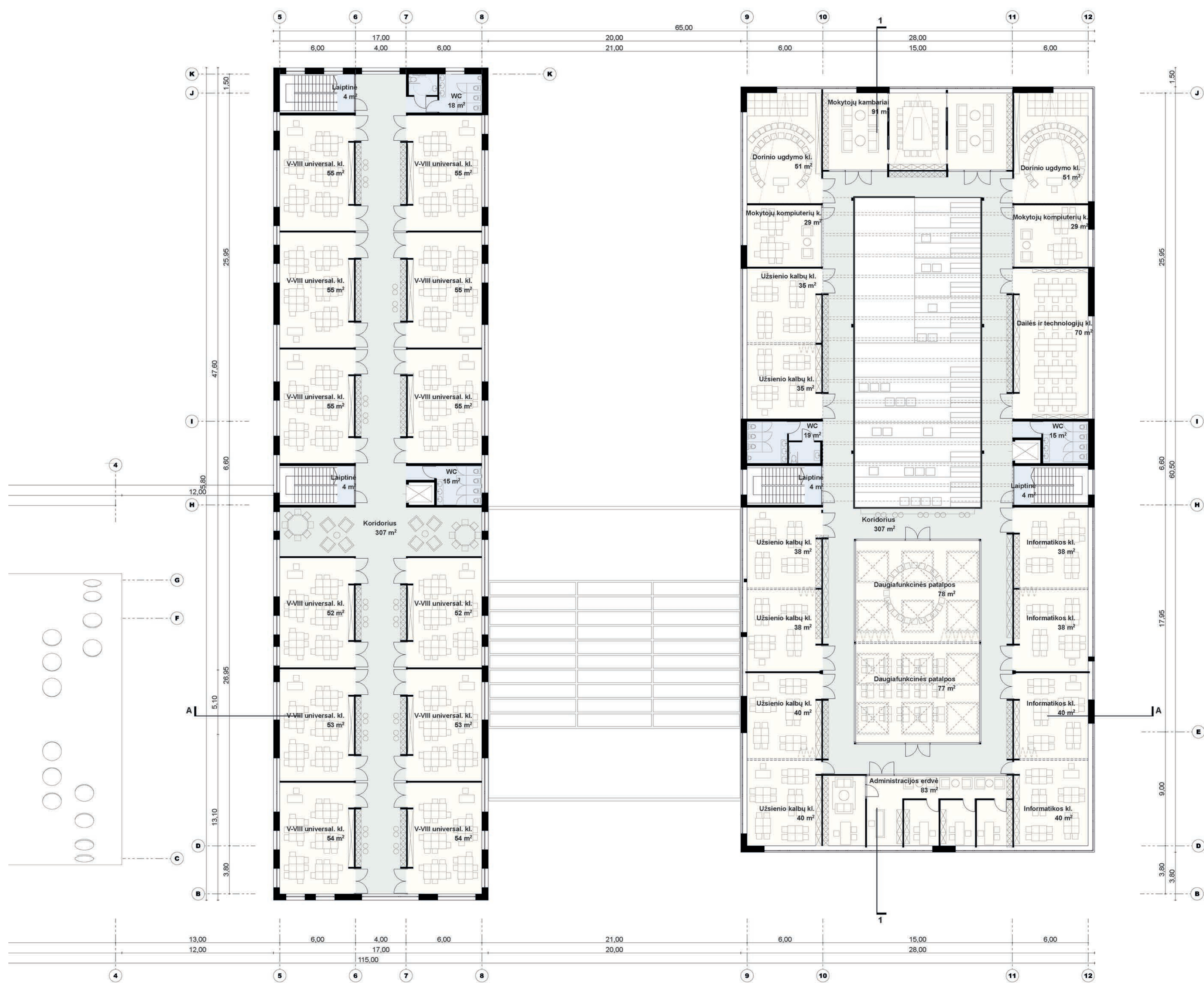
TREČIO AUKŠTO PLANAS M 1:200
