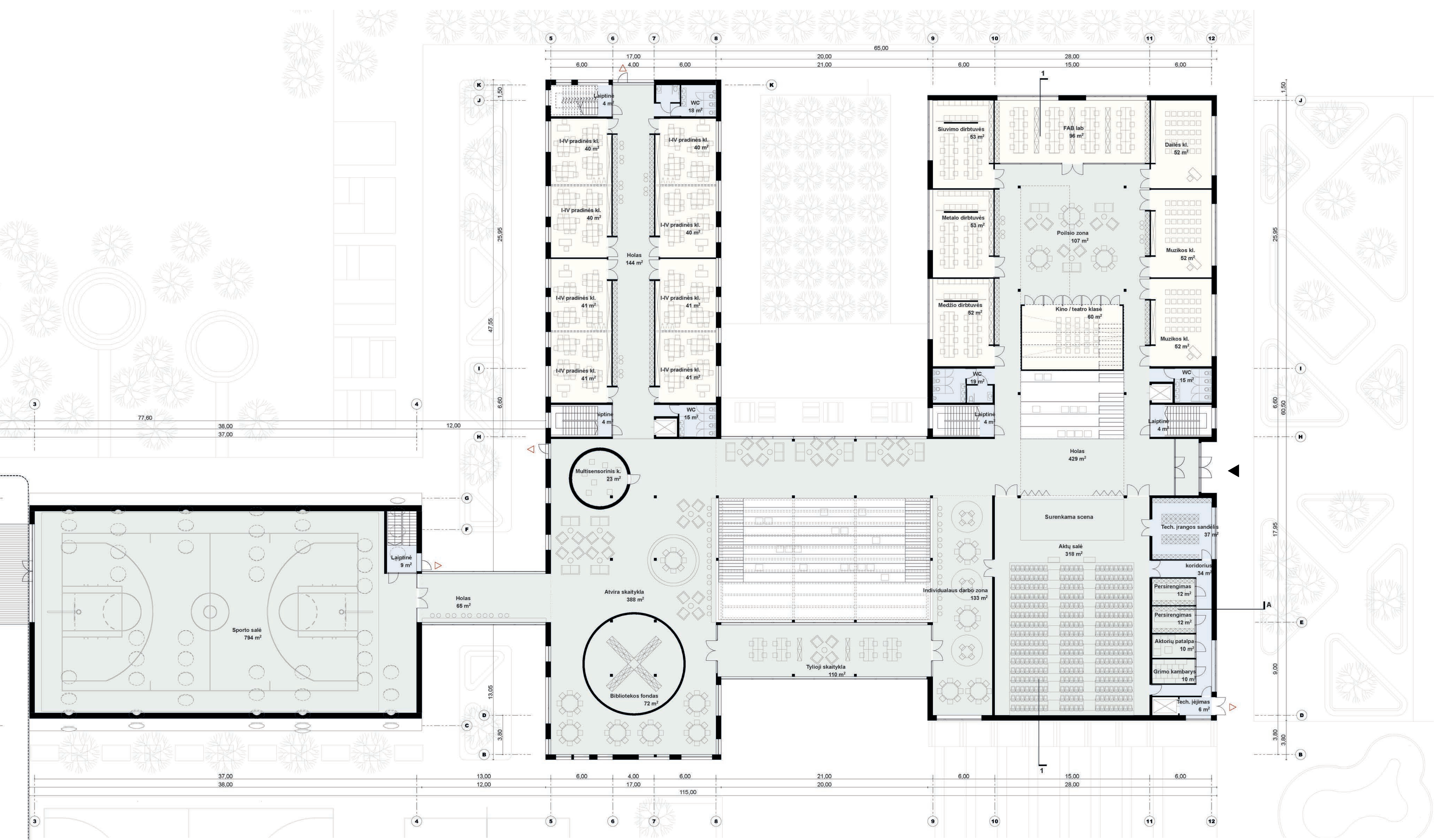
PIRMO AUKŠTO PLANAS M 1:200
