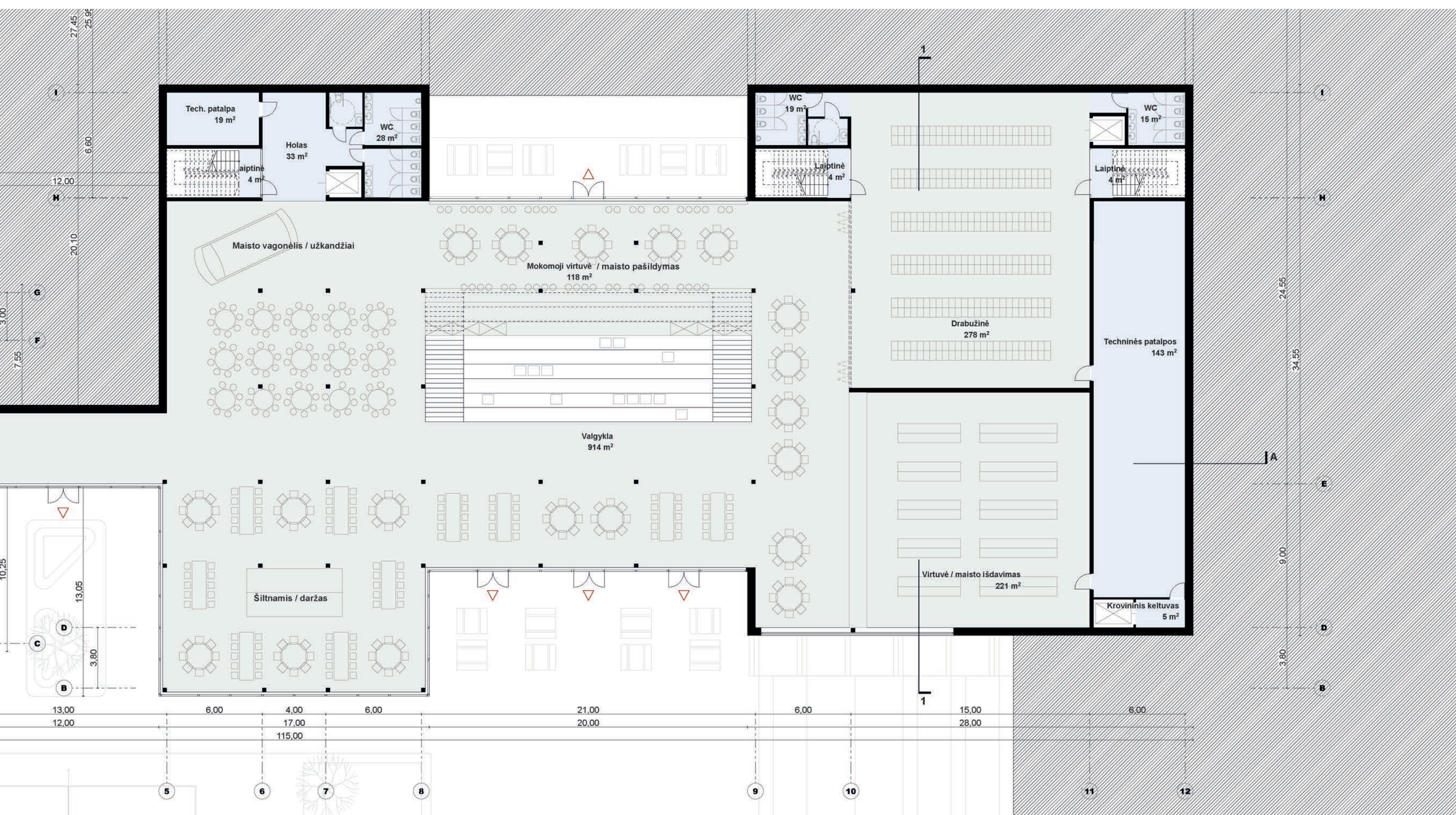
RŪSIO PLANAS M 1:200
