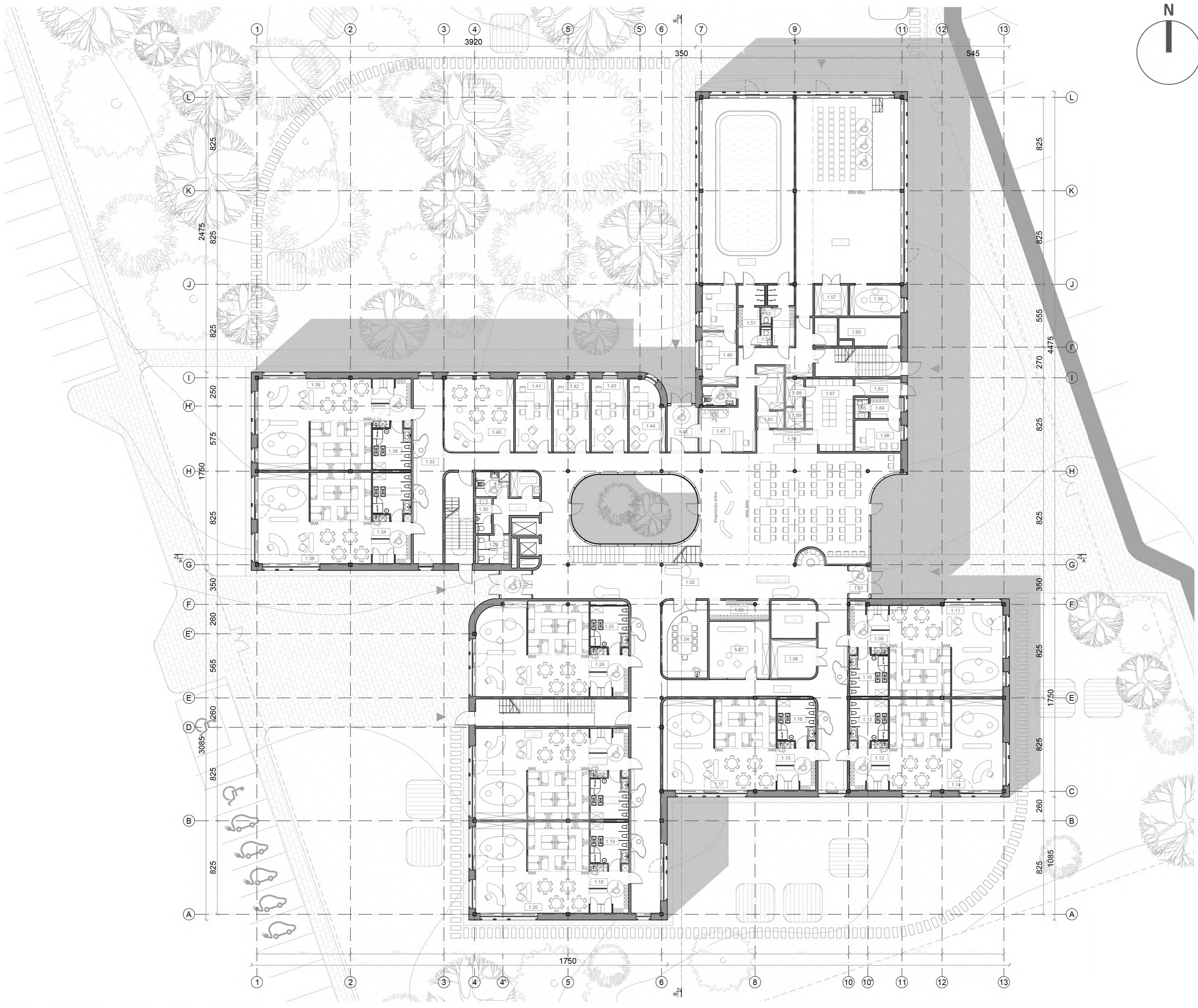
PIRMO AUKŠTO PLANAS, M 1:200
