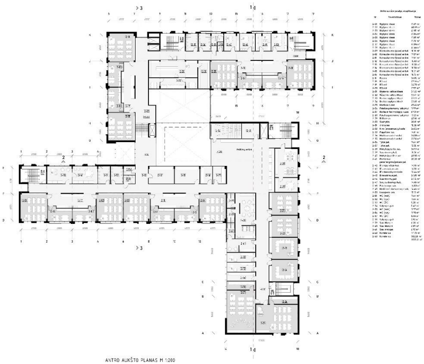
ANTRO AUKŠTO PLANAS M 1:200
