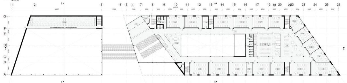
1 PIRMO AUKŠO PLANAS First floor plan M1:250
