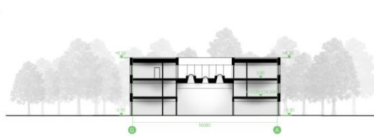
PIŪVIS A-A Section A-A M1:250
