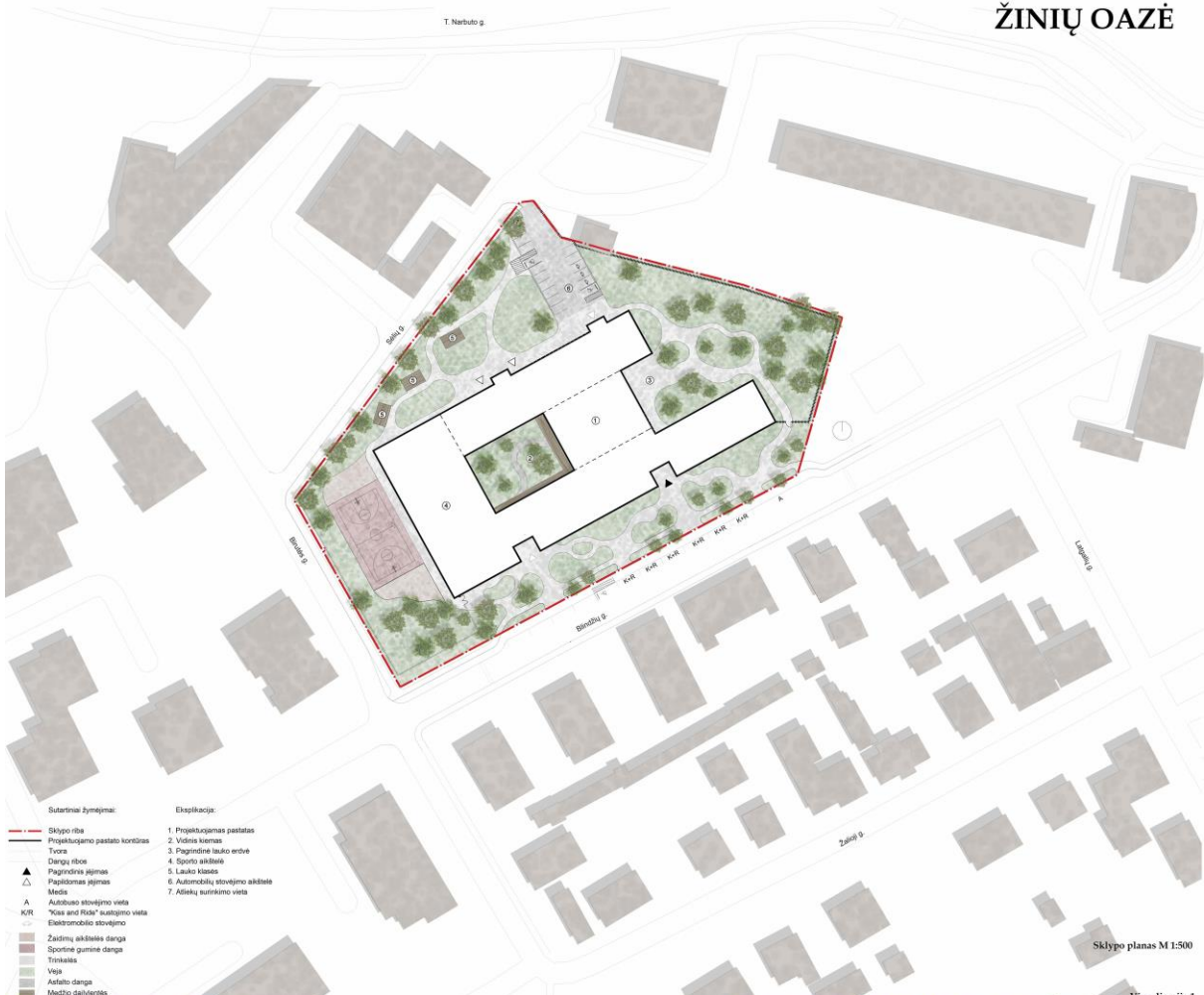
Sklypo planas M 1:500
