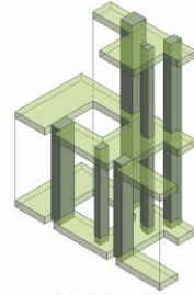
Vertikalių ryšių schema
