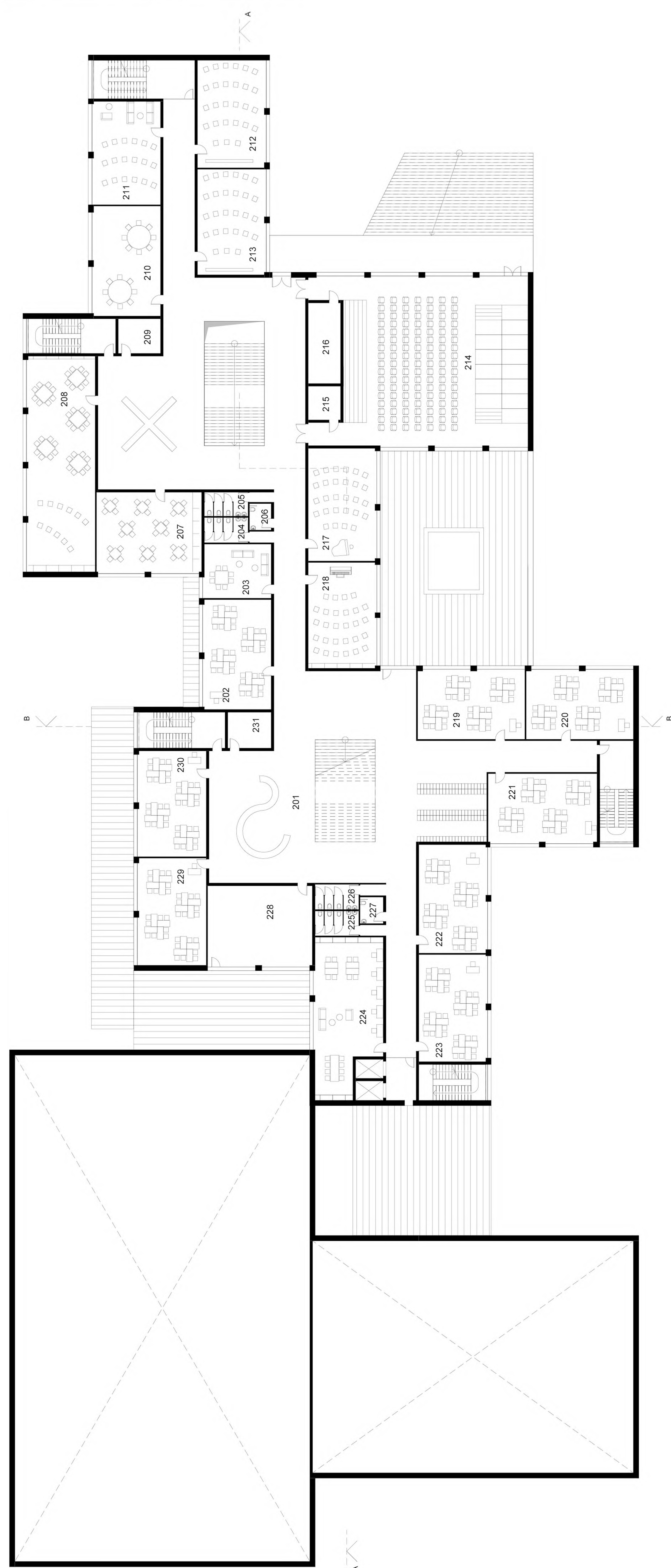
Antro lygio planas, M1:200
